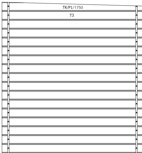
DAK - TOITURE verdeling platen - répartition des panneaux
