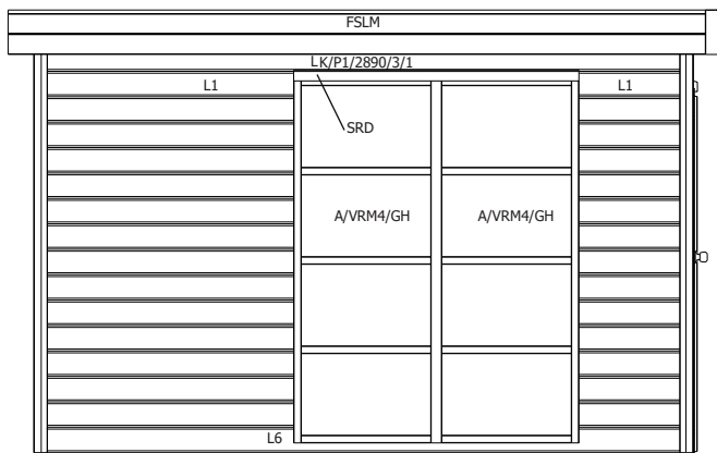
PAROI LATERALE
