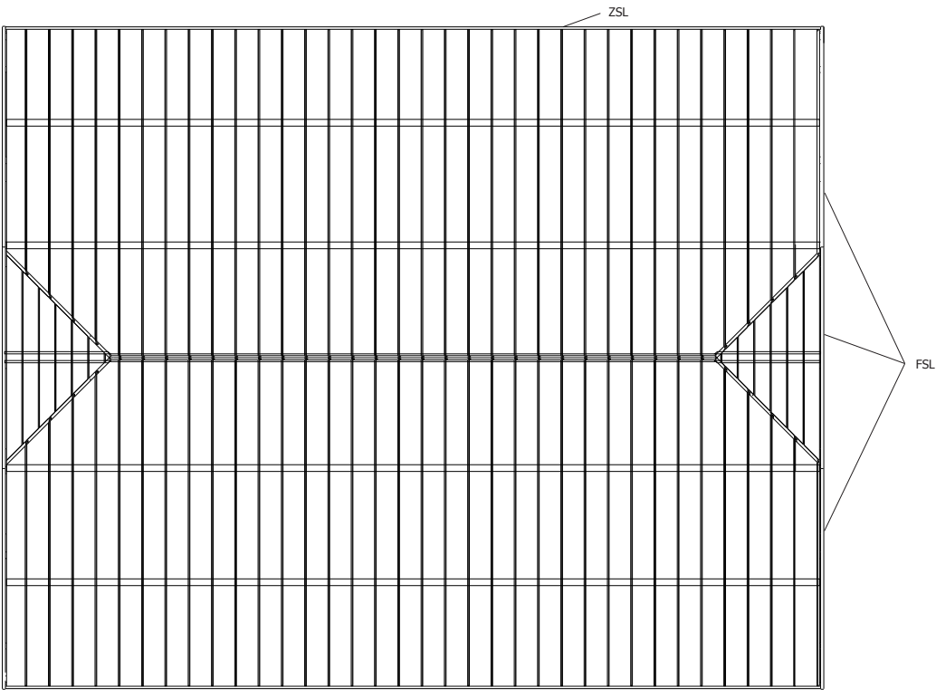
DAK - TOITURE
