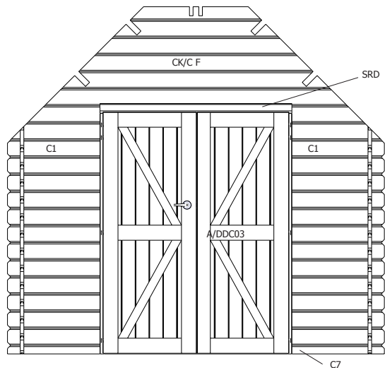
VOORZIJDDE - FACADE
