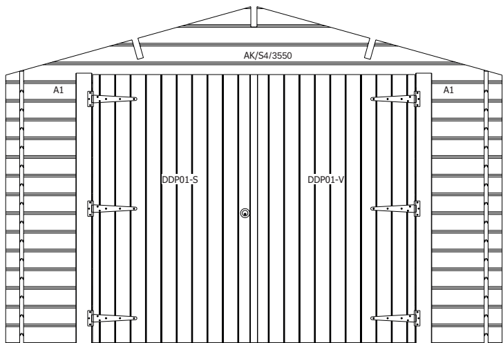
VOORZIJDDE - FACADE
