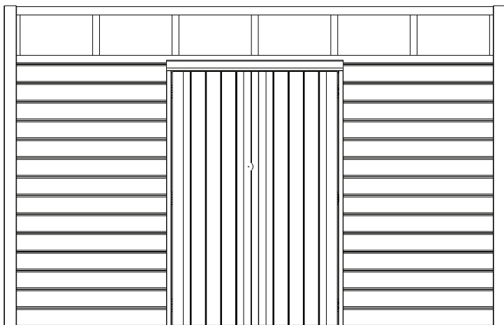
VOORZIJDE - FACADE
