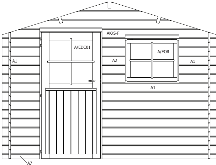
VOORZIJDDE - FACADE
